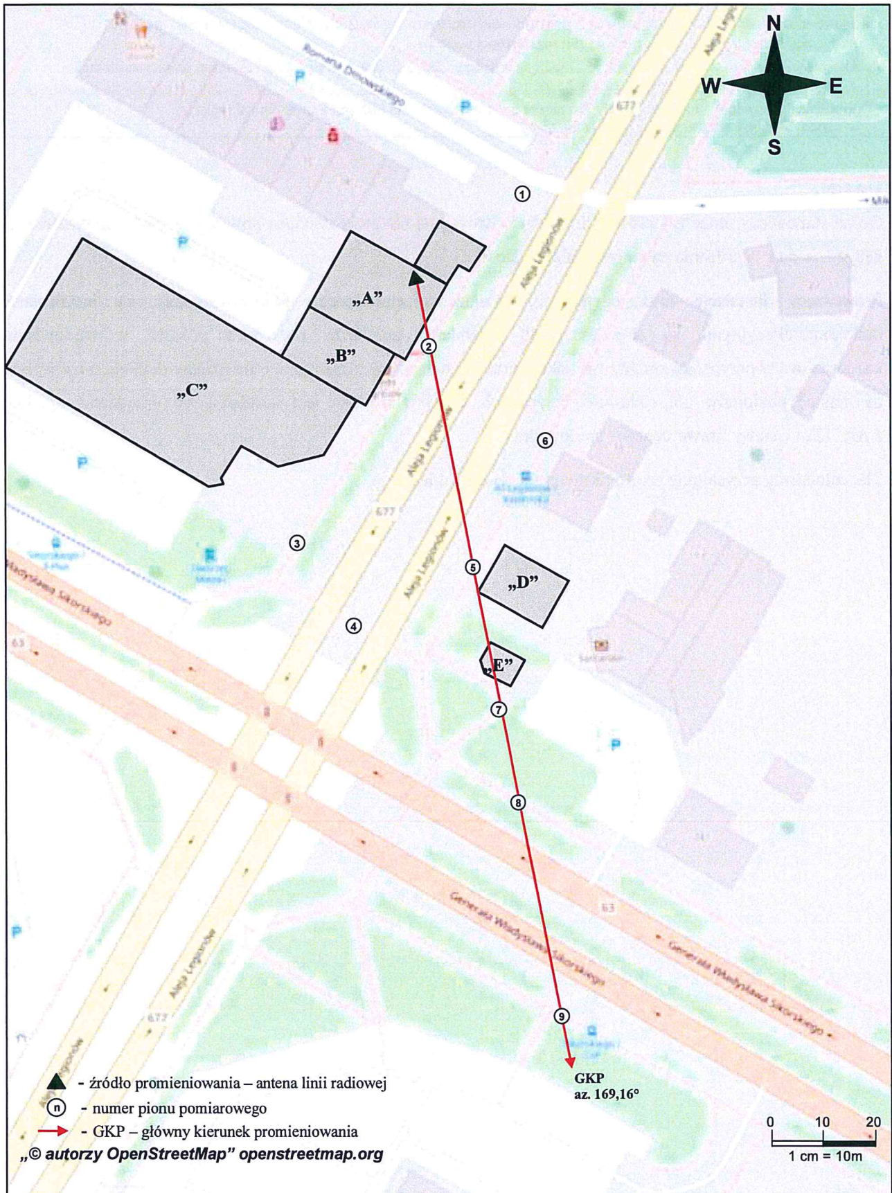
Rys. 1. Usytuowanie punktów i pionów pomiarowych w otoczeniu instalacji radiokomunikacyjnej Stacja Netia LOMZB062-LOMZM00060 Łomża, Aleja Legionów 40
