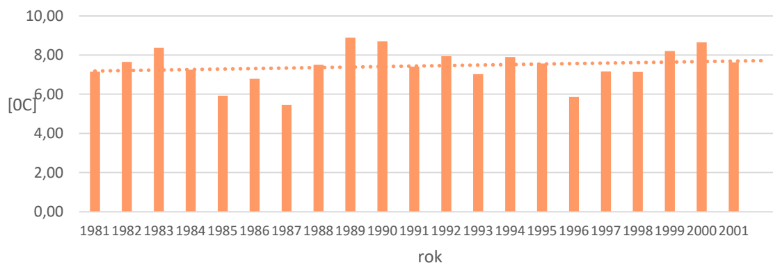
Wykres 15. Średnia dobową temperatura w latach 1981-2002 – stacja Marianowo 46 .
