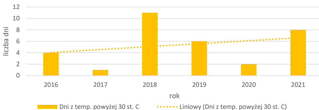
Wykres 11. Liczba dni upalnych (dni z temperaturą maksymalną > 30°C) w latach 2017 - 2021 – stacja Marianowo II 40 .
