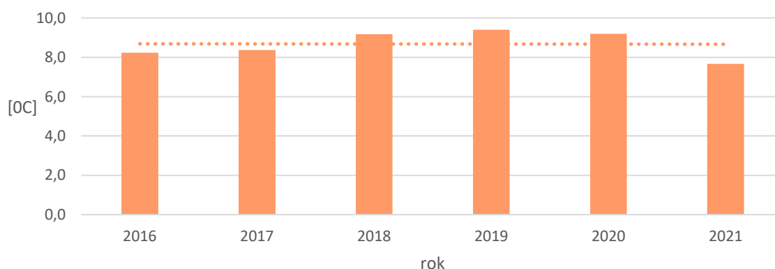
Wykres 16. Średnia dobową temperatura w latach 2016-2021 – stacja Marianowo II 47 .
